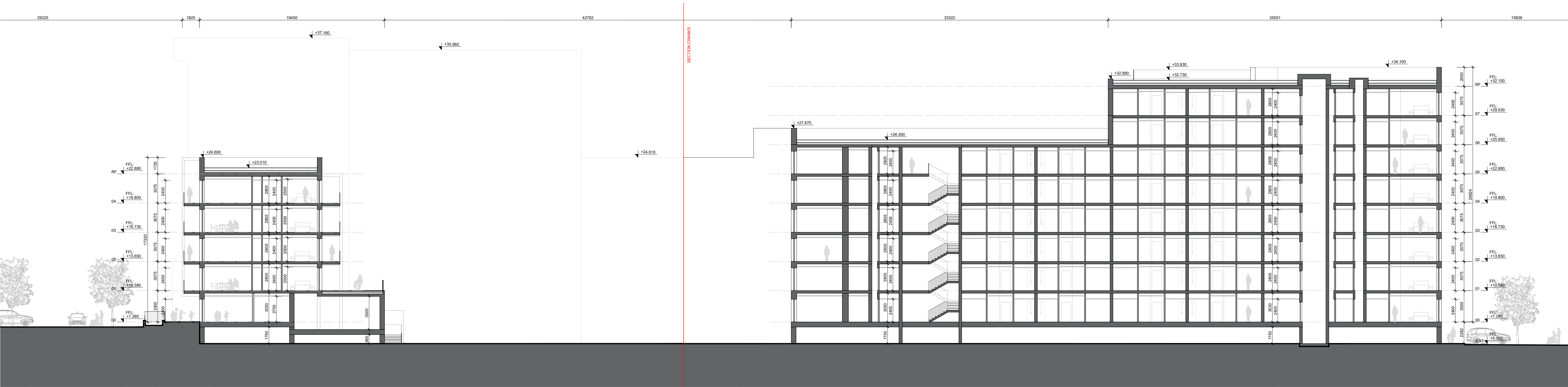
04 SECTION DD 0301 1:200 @A1
