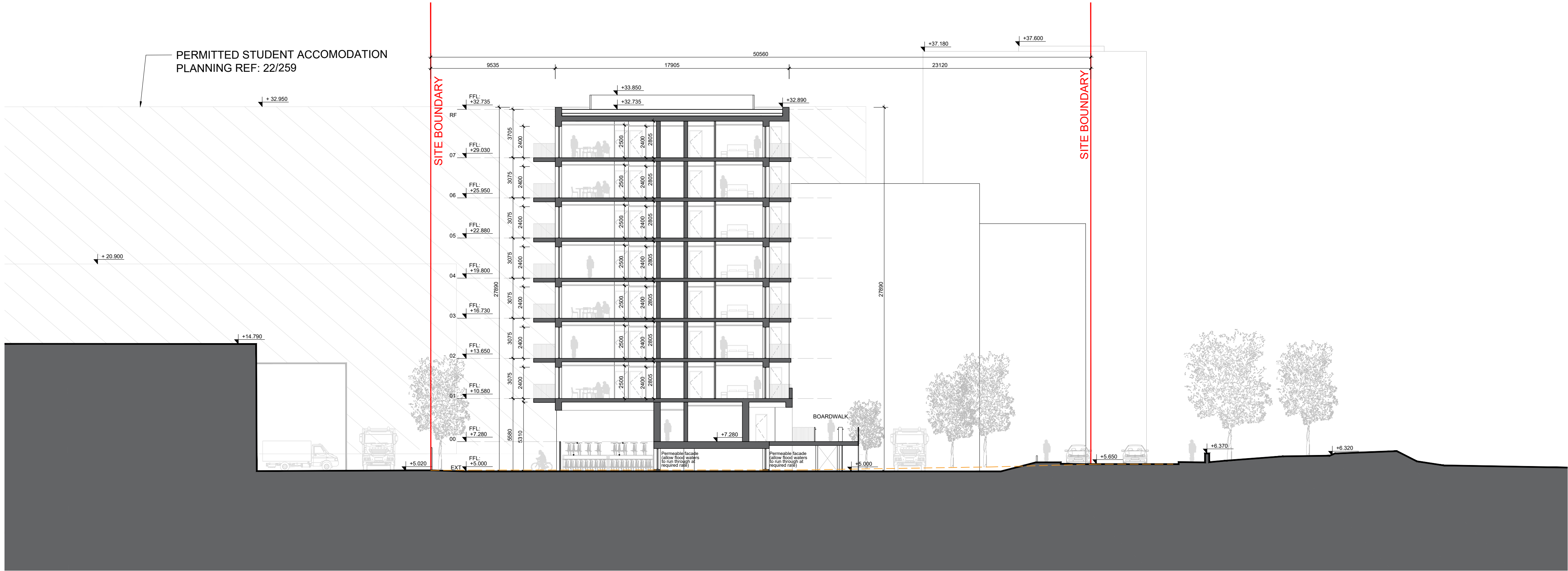
03 SECTION CC 0301 1:200 @A1
